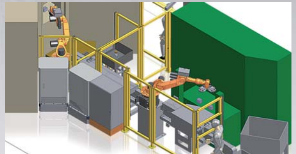
z. B. Verkettung einer Räummaschine und eines Bearbeitungszentrums für PKW-Bremsteile inklusive Staufördersysteme
